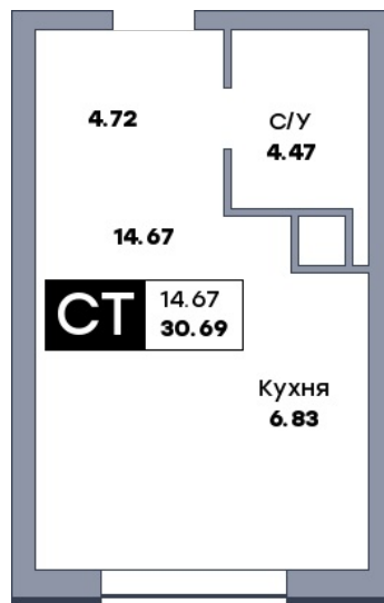
Планировка
