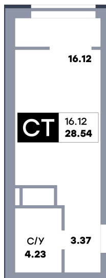
Планировка
