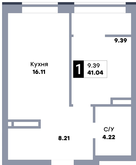
Планировка
