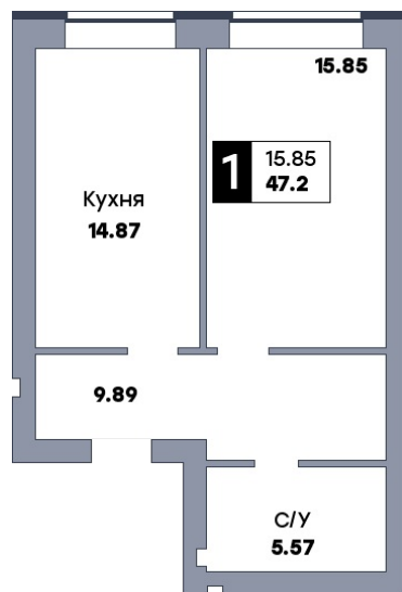
Планировка
