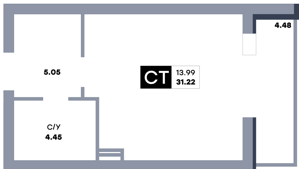
Планировка
