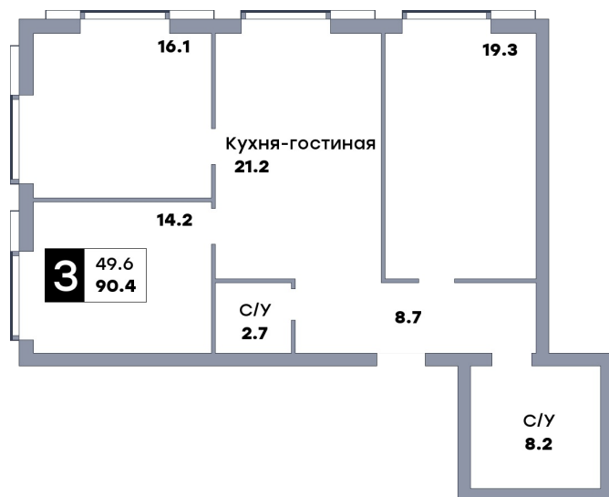
Планировка
