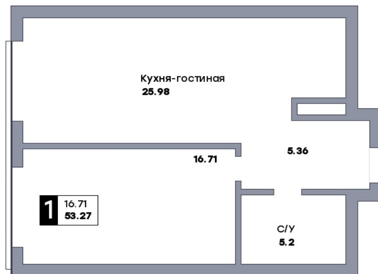
Планировка
