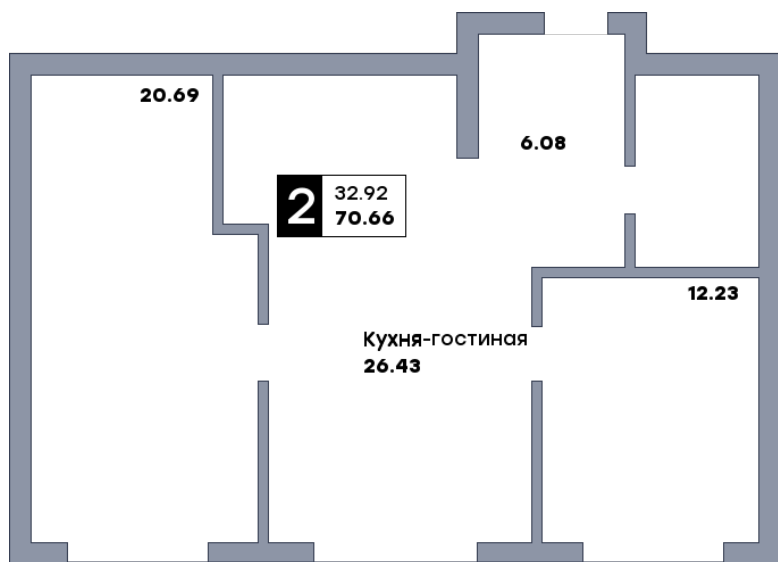
Планировка
