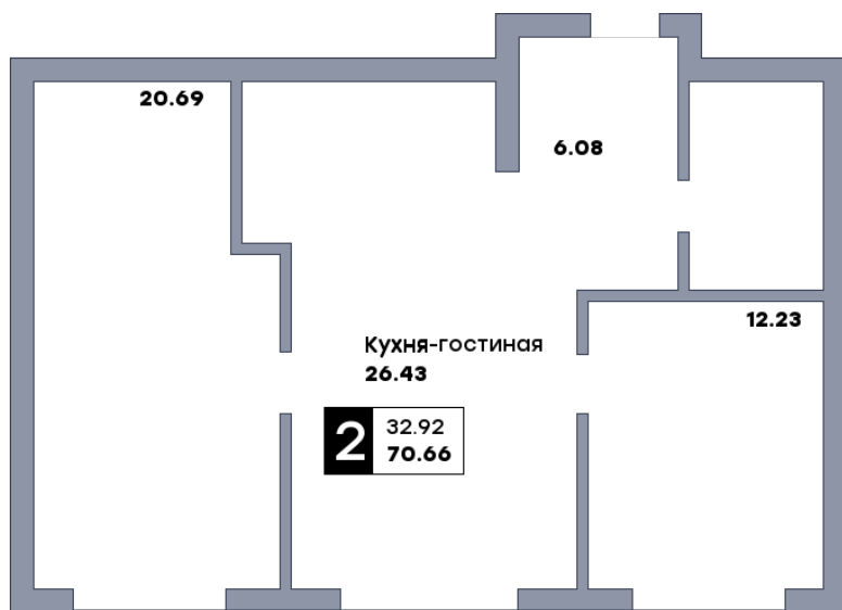
Планировка
