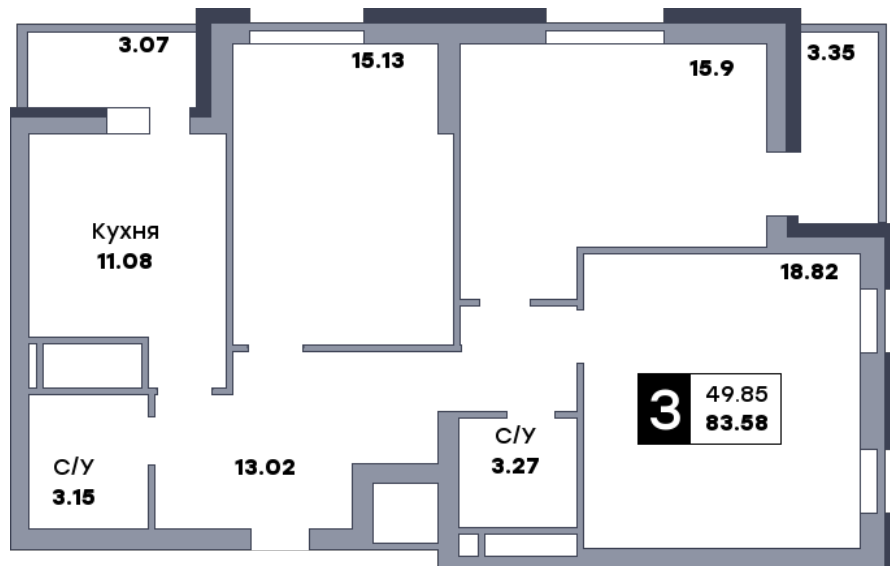
Планировка
