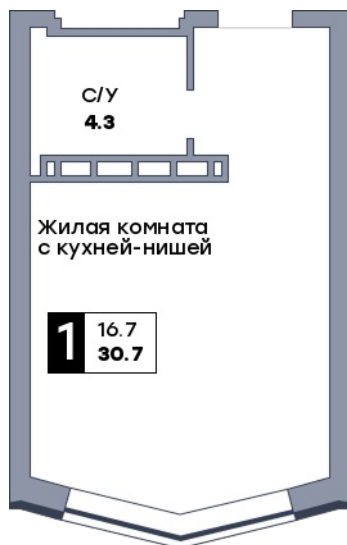
Планировка
