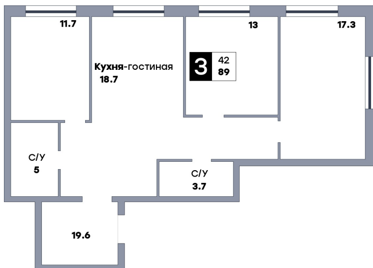
Планировка
